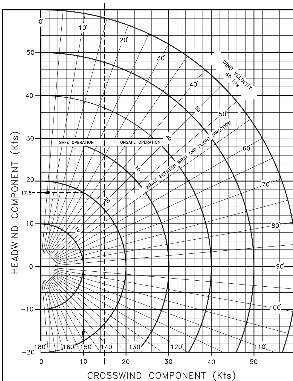
FIG. 5-3. CROSSWIND CHART
