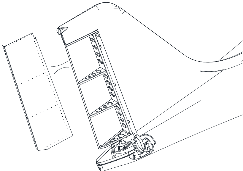
Fig. 7-4. P92 Echo MkII vertical tail and fin
